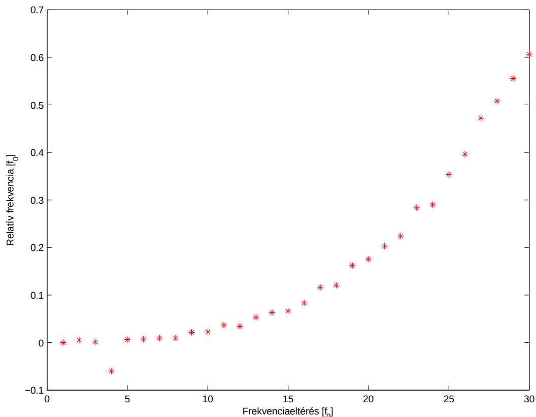
5.3. ábra. Az 1/2-énél pengetett G_2 húr inharmonicitása
