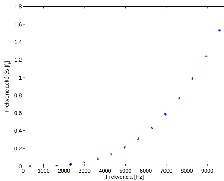
4.8. ábra. A E 4 -es húr inharmonicitása
