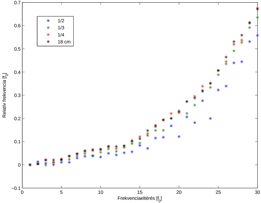
5.4. ábra. A D_2 húr inharmonicitásai a pengetés helyének függvényében
