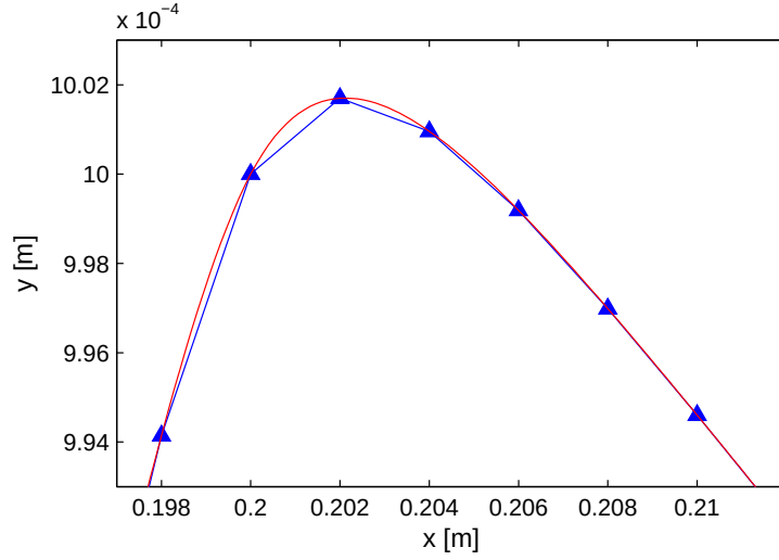
3.4. ábra. Merev húr kezdeti kitérése ideális pengetés esetén a pengetési pozíció közelében. A kék háromszögek a csomópontoknál felvett kitérés értékeket, a piros vonal pedig az alakfüggvények szuperpozícióját kiértékelve kapott eredmény.
