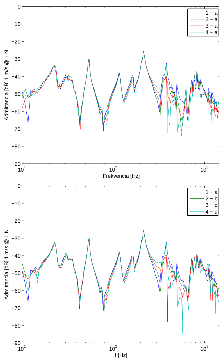
5.6. ábra. A lezárás frekvenciafüggése
