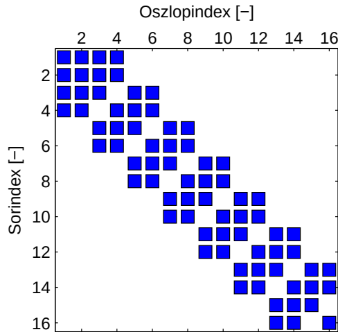
3.3. ábra. Az \mathbf{M} ritka tömegmátrix első néhány sorának és oszlopának szerkezete
