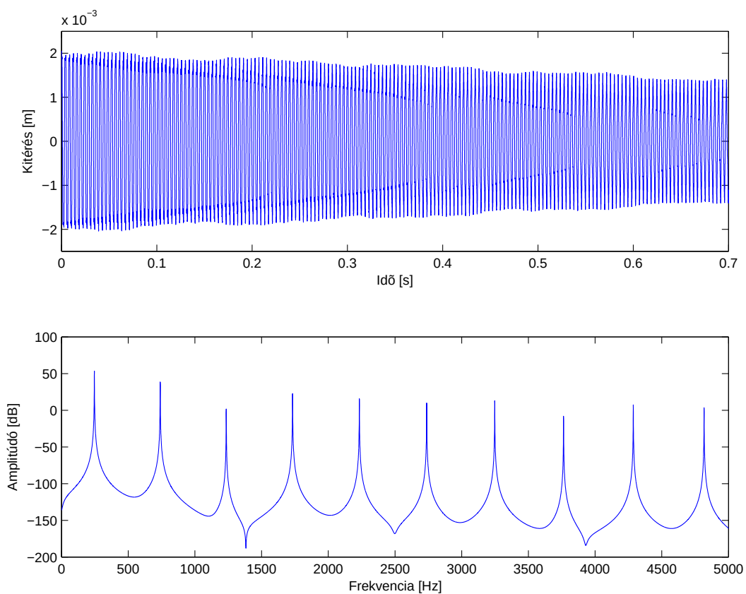
4.7. ábra. A B 3 -as húr idő-, és frekvenciatartományban
