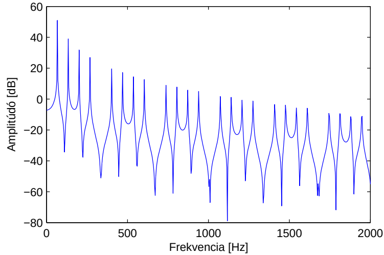
4.3. ábra. Egy pont kitérésének spektruma az ideális, csillapítatlan esetben
