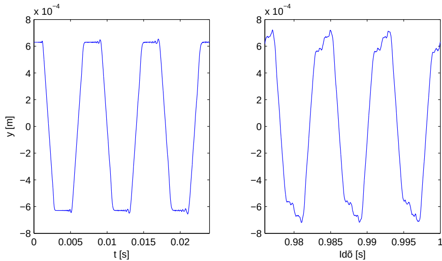
4.5. ábra. A merev húr egy pontjának kitérése, a jelalak elváltozása a diszperzió hatására. Bal: az első néhány szimulált periódus jelalakja. Jobb: jelalak a szimulált időtartam végén.
