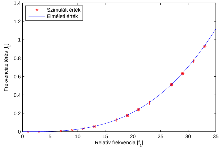
4.6. ábra. Inharmonicitás a diszperz húrban, az elméleti és szimulált módusfrekvenciák összehasonlítása
