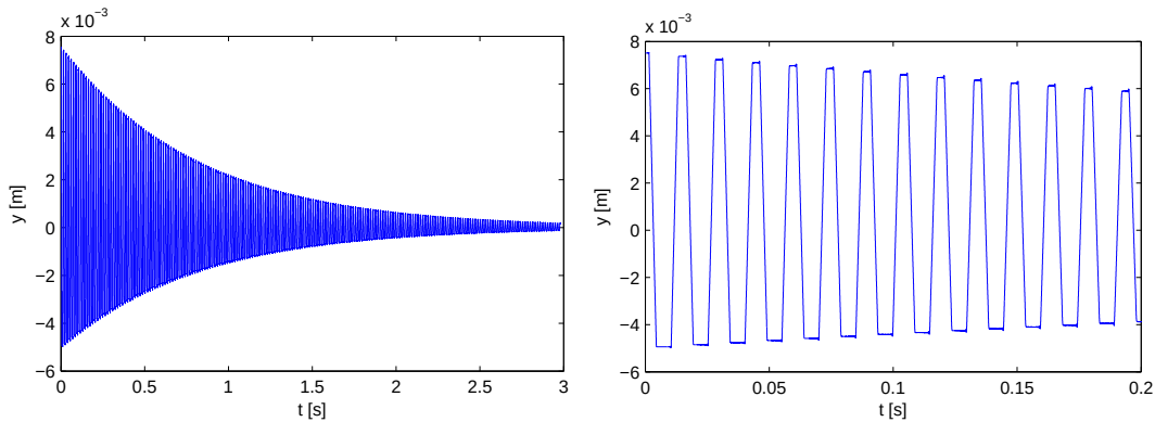
4.4. ábra. A csillapított húr egy pontjának kitérése az idő függvényében. Bal: a teljes szimulált időfüggvény. Jobb: az első néhány periódus közelről.
