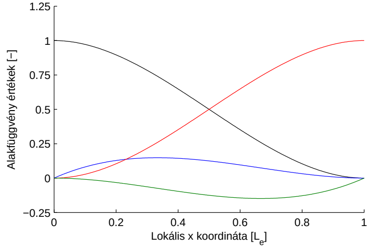
3.2. ábra. A nemideális modell egy elemhez tartozó négy alakfüggvénye
